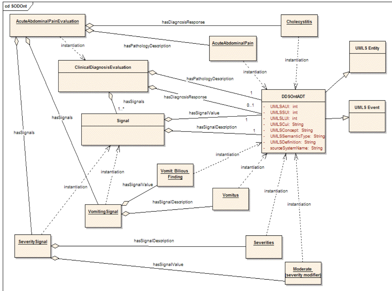
Figura 4 - Ontologia DDSOnt
