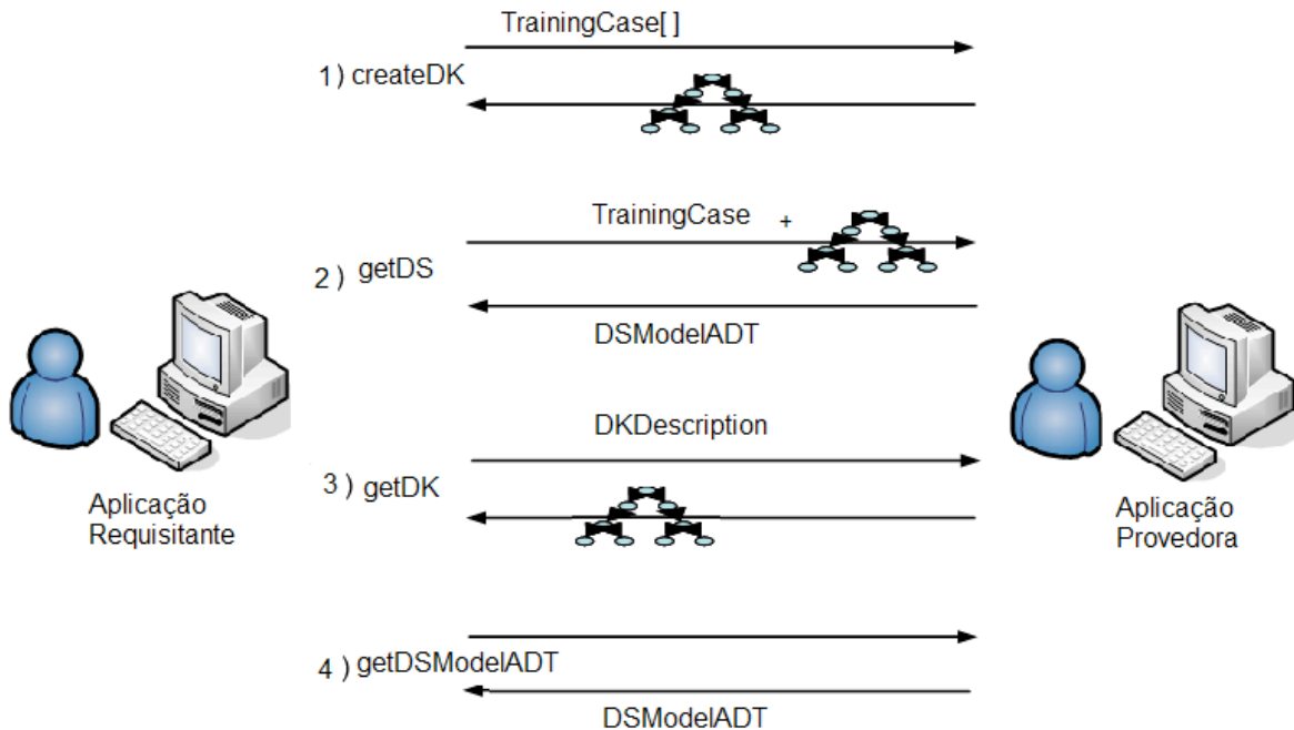
Figura 2 - Especificação DSModelWs
