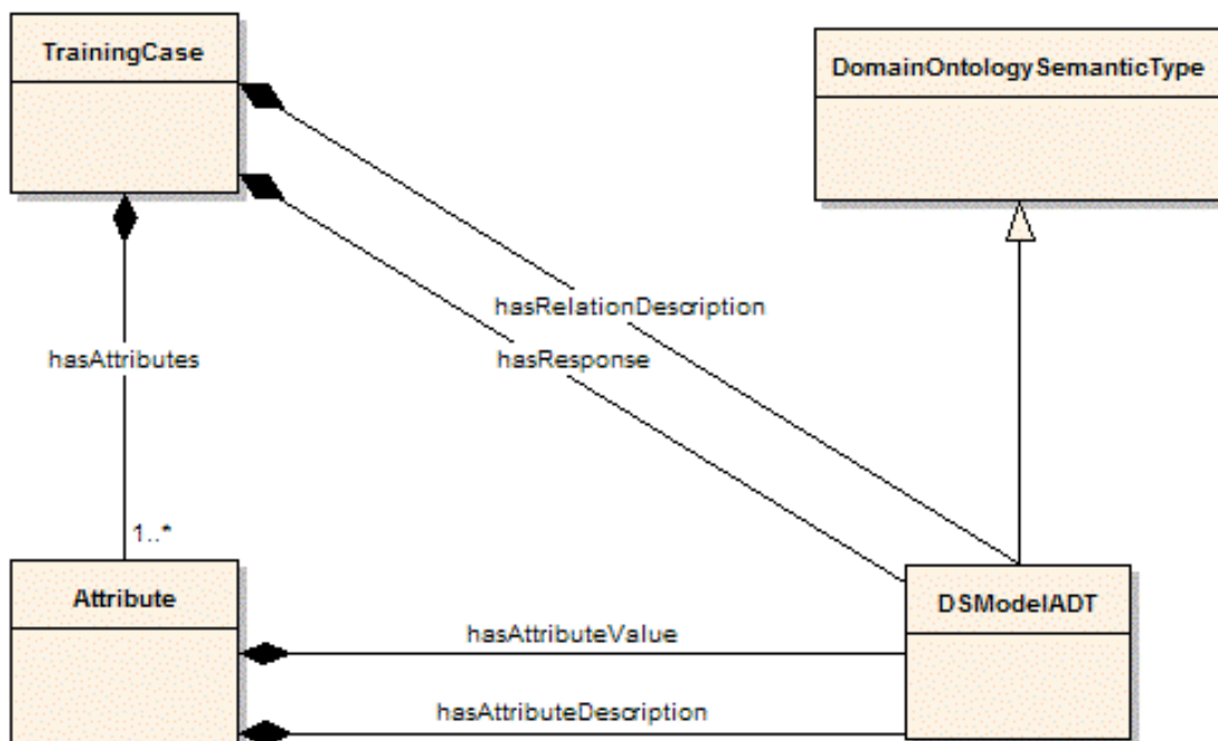
Figura 1 - Modelo DSModel
